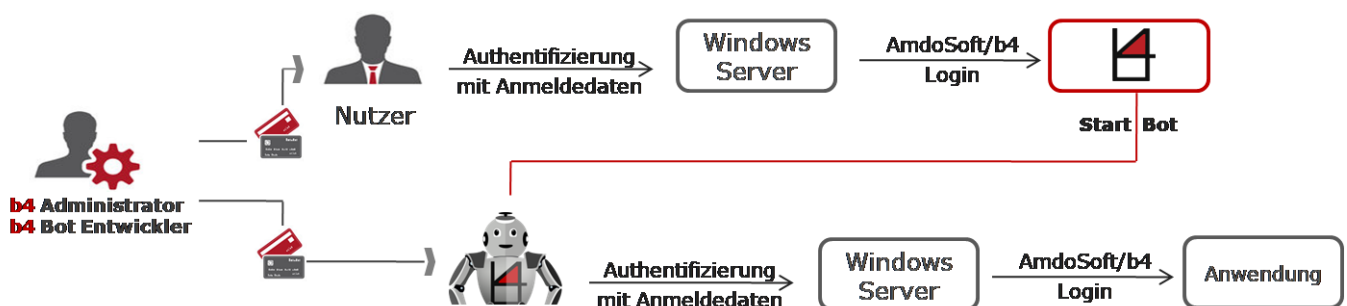
Abbildung 5: Unbeaufsichtigte Automatisierung
